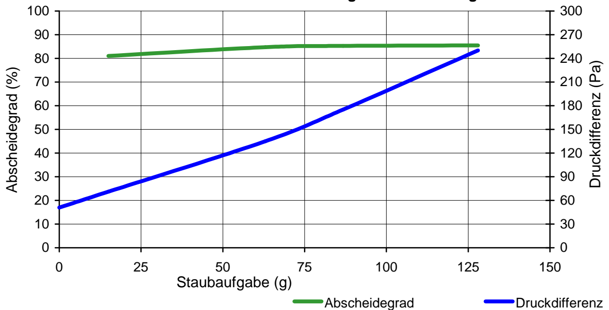
Druckdifferenz und Abscheidegrad zu Staubaufgabe
